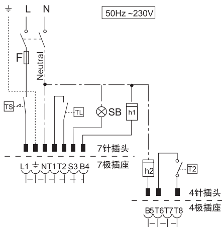
燃烧器电气连接
