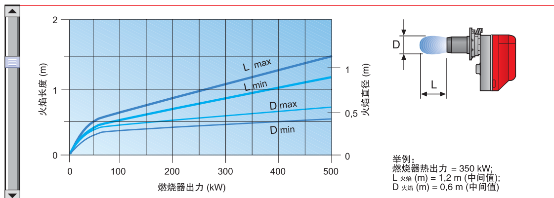
燃烧头
