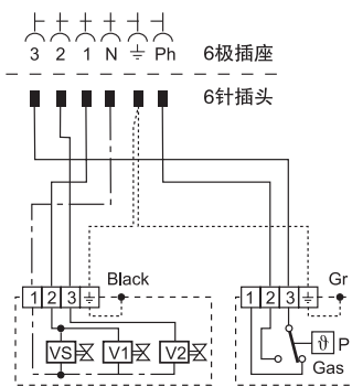
燃气阀组电气连接
